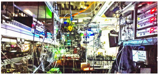
Computación cuántica |
